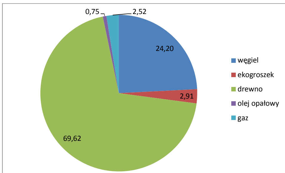
Rysunek 12. Udział paliw w zużyciu energii na cele ogrzewania i przygotowania posiłków w gospodarstwach domowych w gminie Nur
