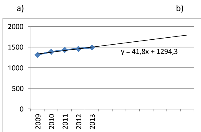
Rysunek 18. Prognoza zmiany liczby pojazdów ciężarowych oraz osobowych w gminie Nur w latach 2014-2020 , a) samochody osobowe, b) samochody ciężarowe
