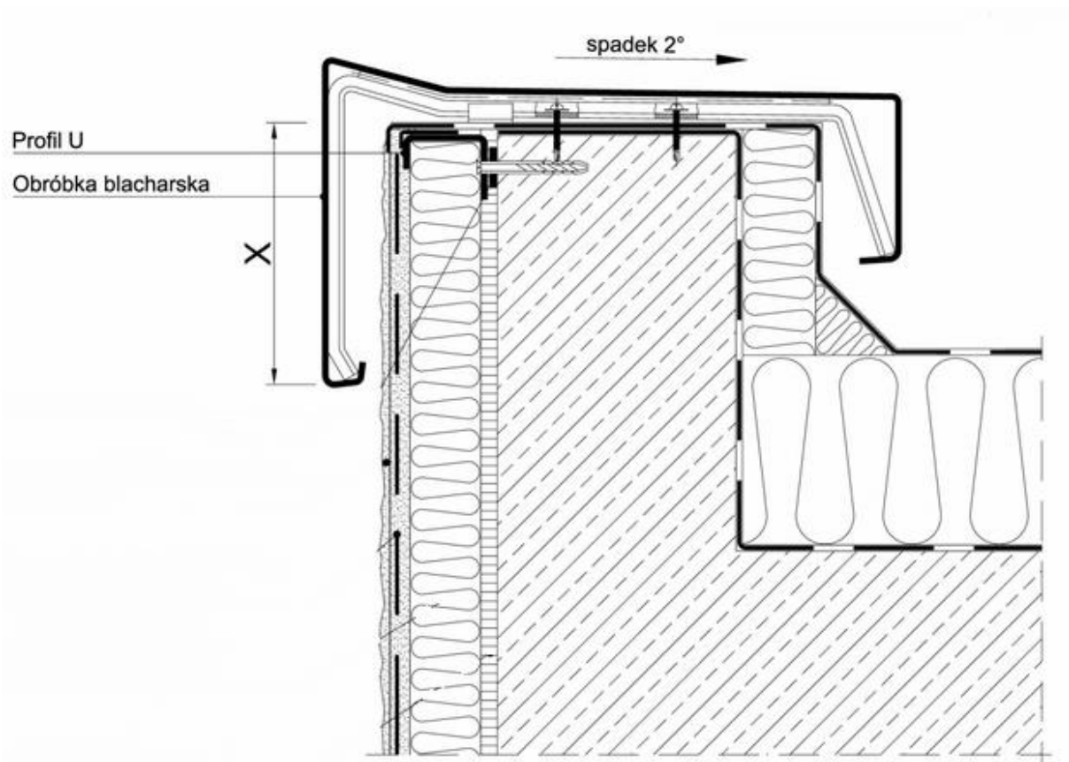
Rys. 1 Przykład wykonania detalu połączenia stropodachu ze ścianą konstrukcyjną. Szczegóły do ustalenia z Inwestorem (ocieplenie ściana konstrukcyjnych nie wchodzi w zakres inwestycji).
