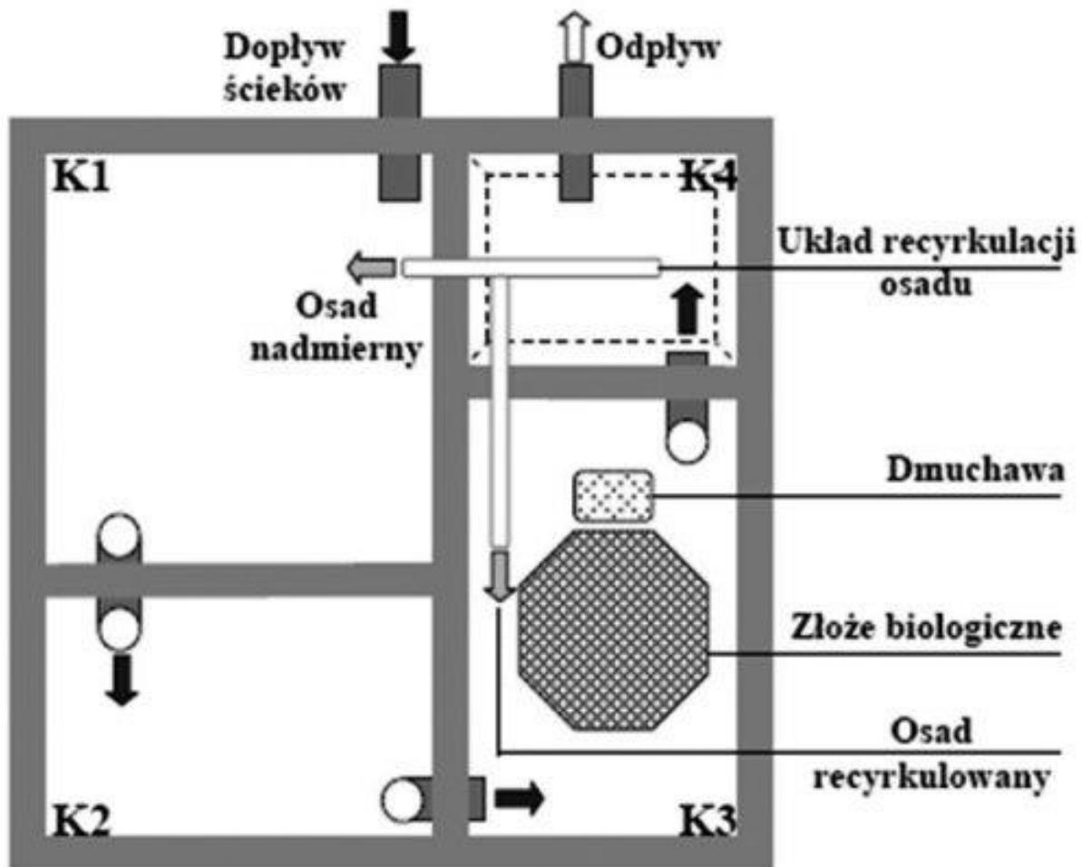
Rys. nr 5. Oczyszczalnia przydomowa hybrydowa.
