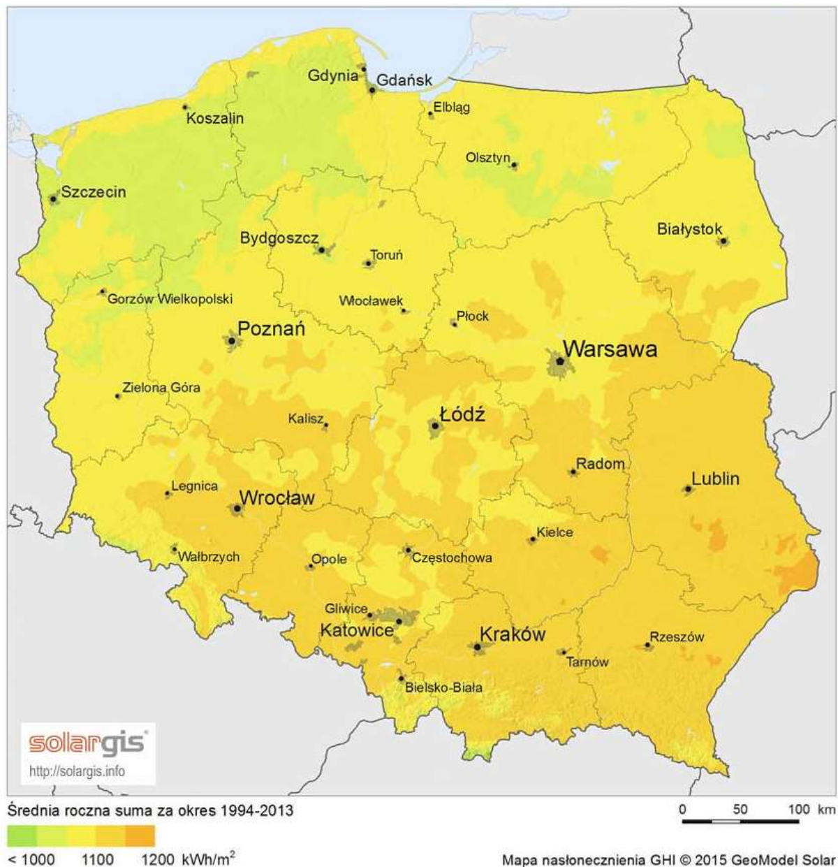
Mapa 6. Poziom nasłonecznienia w Polsce
