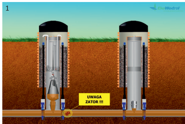
Sposób płukania odcinka rurociągu, w którym powstał zator. (Prezentacje multimedialne dostępne są na stronie internetowej www.ekowodrol.pl )
