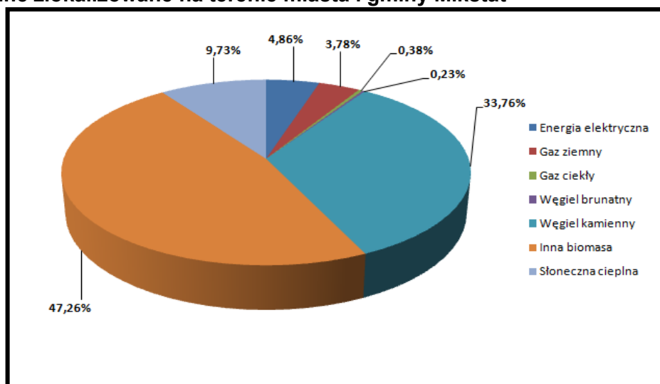
Rys.6 Szacunkowy udział zużycia poszczególnych nośników energii przez budynki mieszkalne zlokalizowane na terenie miasta i gminy Mikstát
