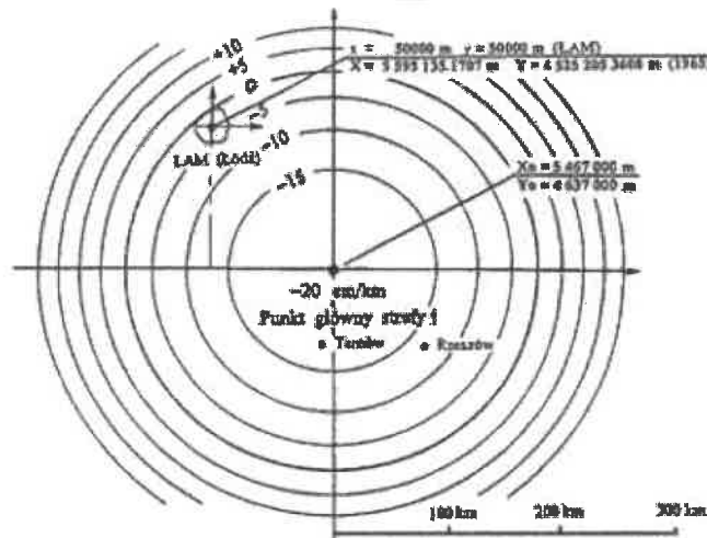
Rys. 4. Położenie układu lokalnego miasta Łodzi (ŁAM) na tle izolini zniekształceń liniowych w strefie I układu 1965, obrazujące zmienność skali w transformacji xy_{\text{LOK}} \Leftrightarrow xy_{65}
