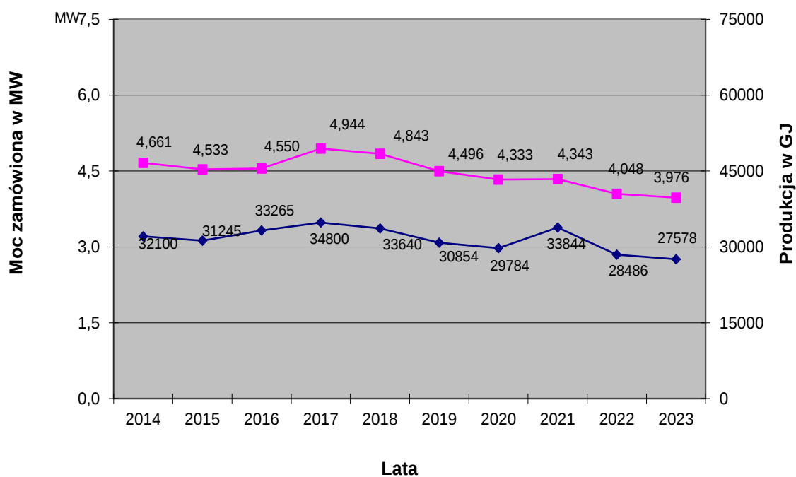
Wykres 4. Porównanie mocy zamówionej ze sprzedaną energią cieplną w latach 2014 - 2023
