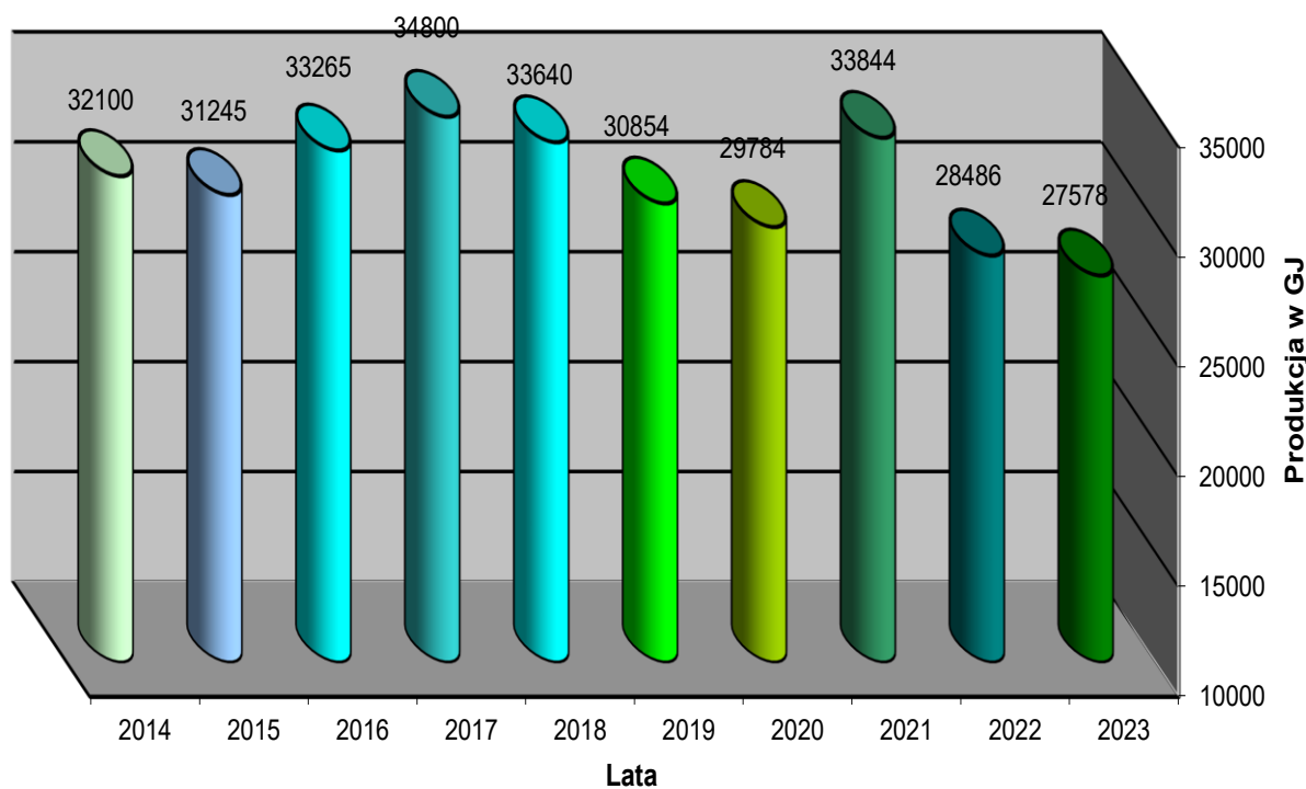
Wykres 3. Wielkość sprzedanej energii cieplnej w latach 2014 - 2023
