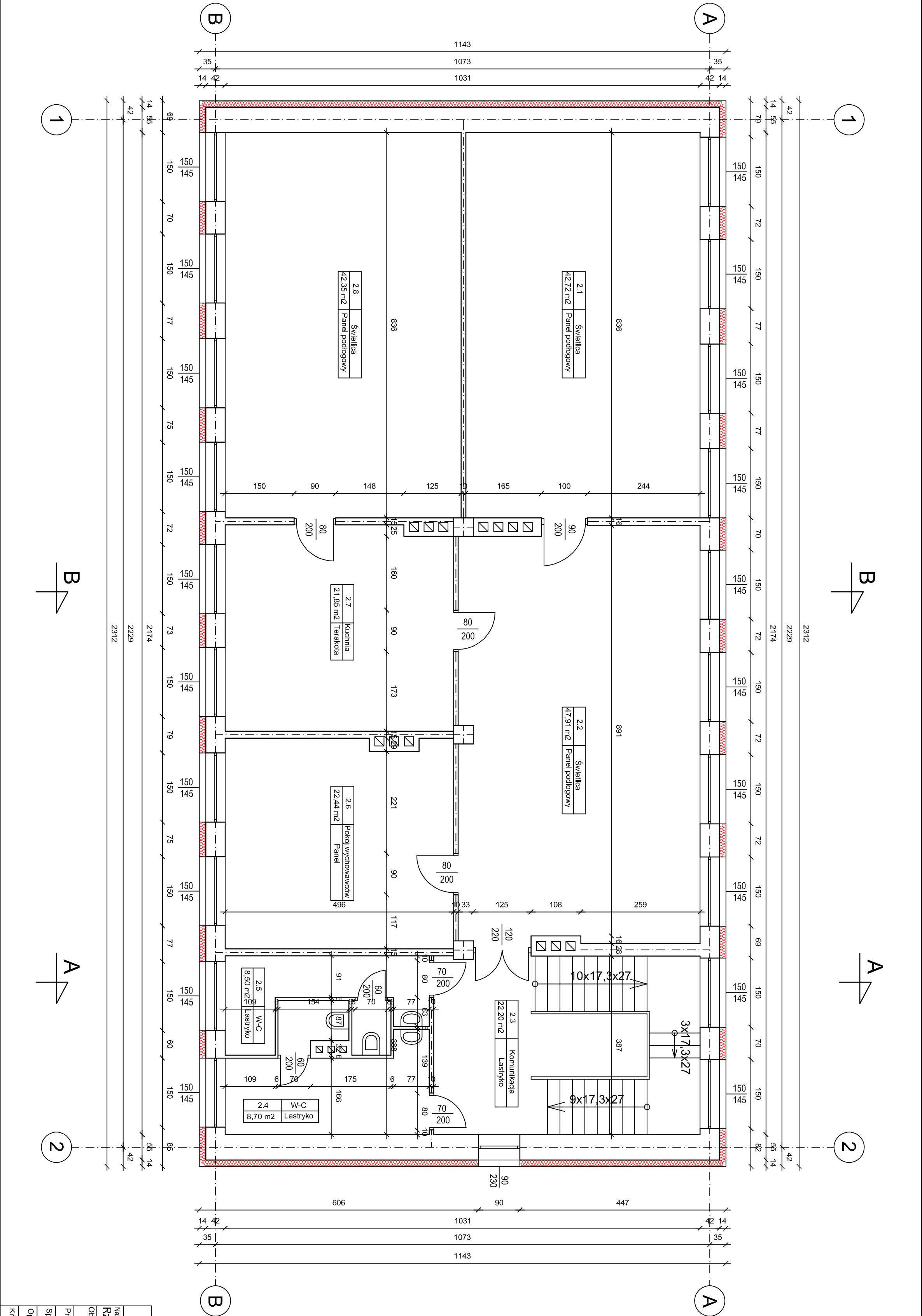
Rzut piętra
