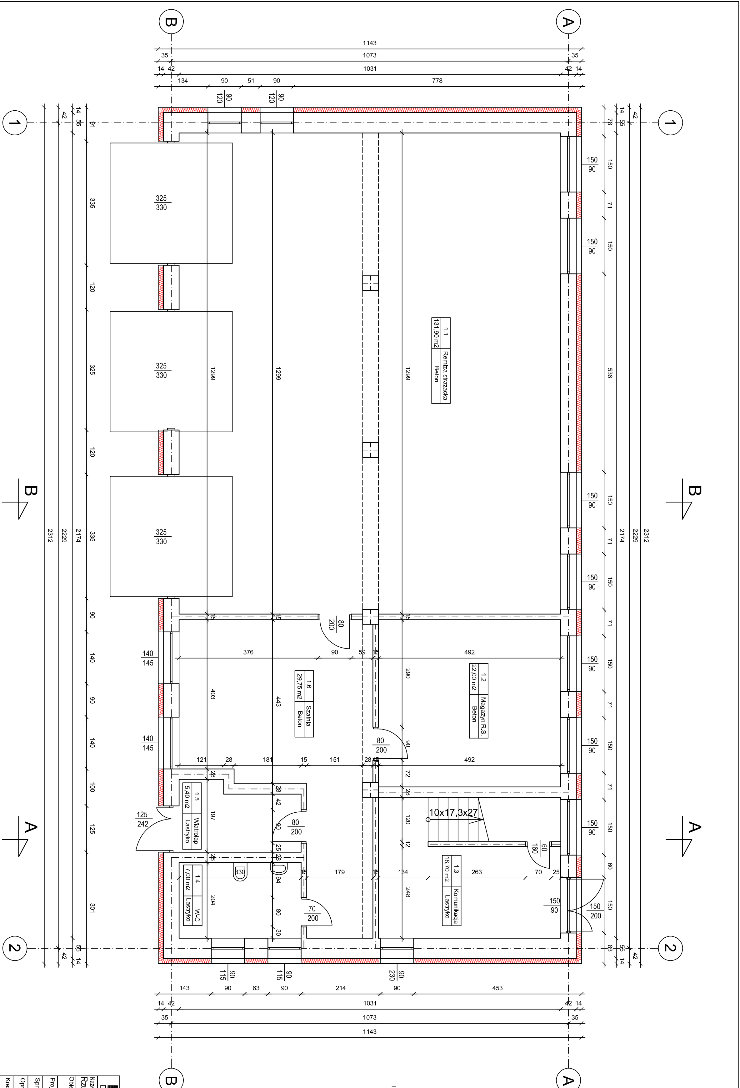
Rzut parteru 1:50
