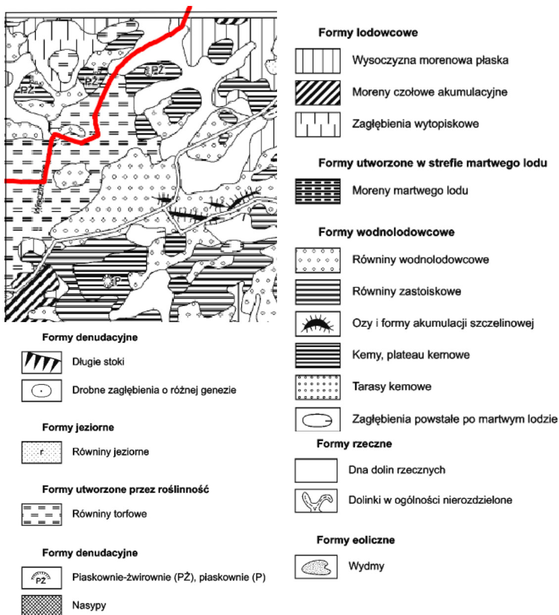
Rysunek 12. Szkic geomorfologiczny w południowo - wschodniej części Gminy Wieczfnia Kościelna Źródło: Objasnienia do Szczegółowej Mapy Geologicznej Polski 1:50 000, Arkusz Grudusk (329) Tablica I
