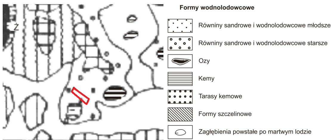
Rysunek 9. Szkic geomorfologiczny dla obszaru mpzp Źródło: Objąsnienia do Szczegółowej Mapy Geologicznej Polski 1:50 000, Arkusz Janowo (290) Tablica I
