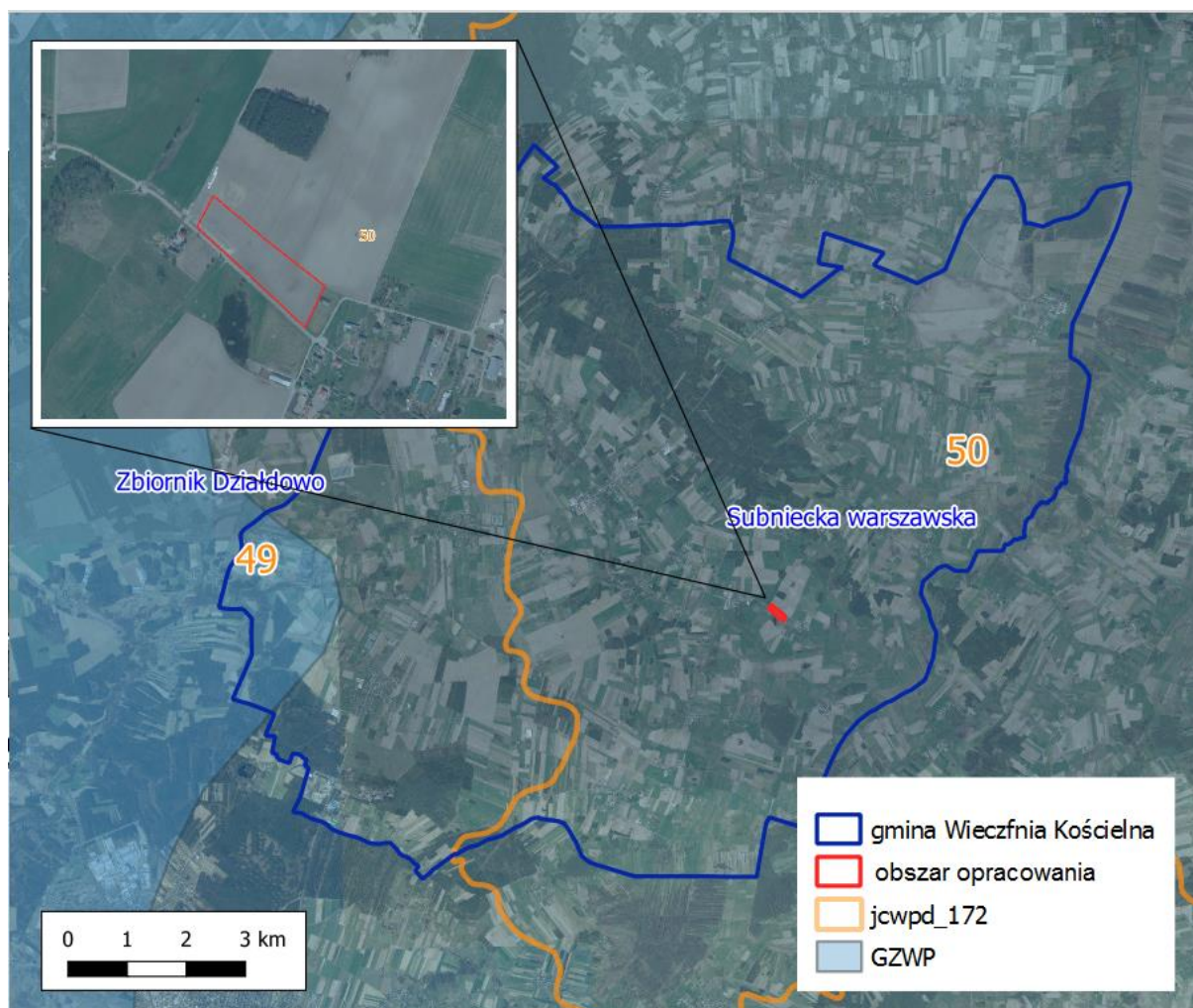
Rysunek 15. Lokalizacja GZWP oraz JCWPd na terenie objętym opracowaniem
