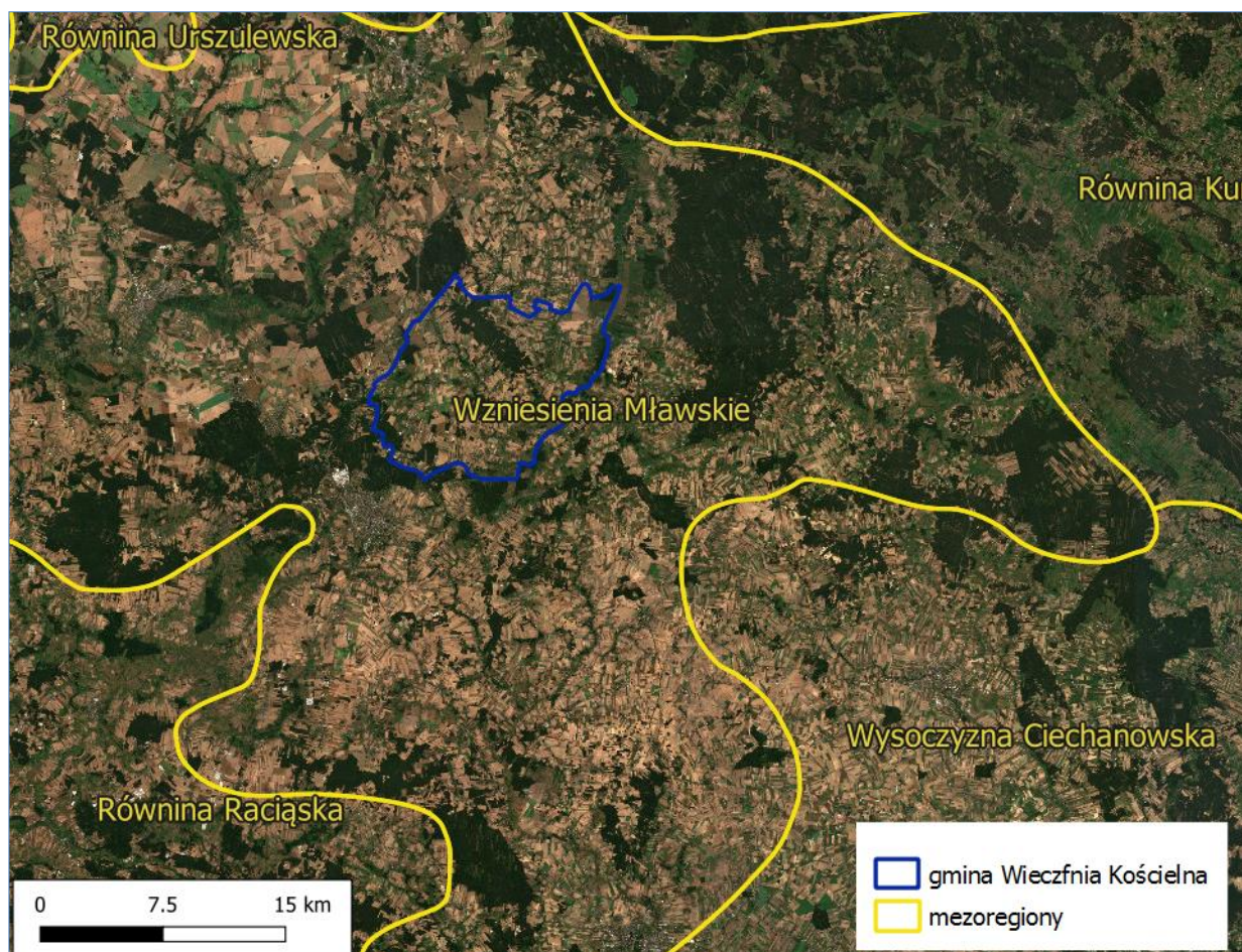
Rysunek 6. Regiony fizyczno-geograficzne na terenie Gminy Wieczfnia Kościelna Źródło: opracowanie własne na podstawie danych pochodzących z Centralnej Bazy Danych Geologicznych
