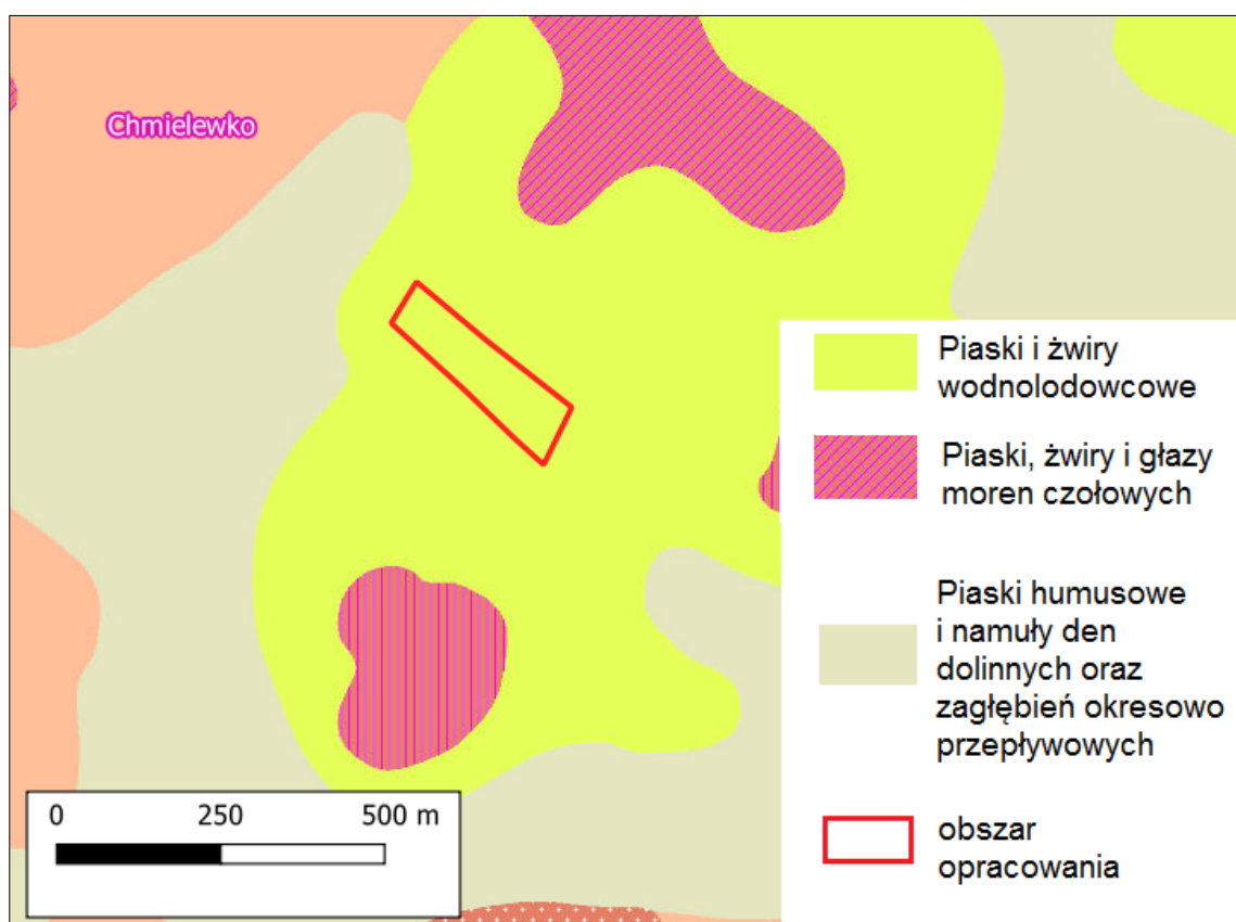
Rysunek 10. Szczegółowa Mapa geologiczna Polski Źródło: opracowanie własne na podstawie Arkusza Janowo (290)
