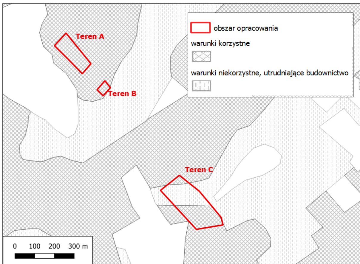
Rysunek 9. Warunki podłoża budowlanego
