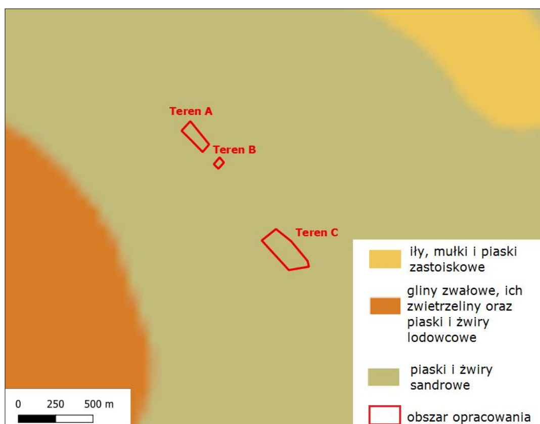
Rysunek 6. Mapa geologiczna dla obszaru opracowania mpzp. Źródło: www.bazagis.pgi.gov.pl
