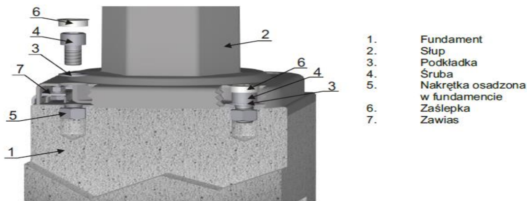
Szczegół montażu zabezpieczenia
