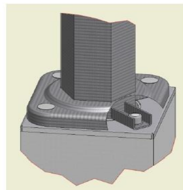
Szczegół węzła po zmontowaniu
