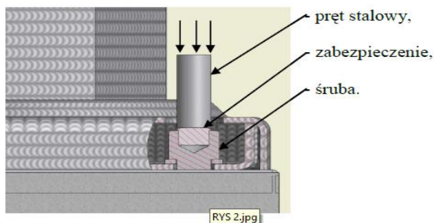
Szczegół montażu zabezpieczenia
