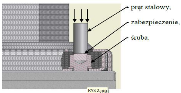
Szczegół montażu zabezpieczenia
