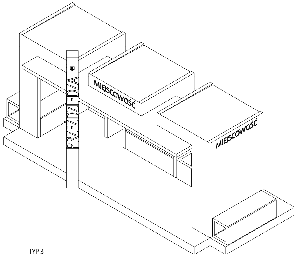
TYP 3 SŁUP Z ROZKŁADEM JAZDY +2 MODUŁY PODSTAWOWE +MODUŁ ROZSZERZAJĄCY
