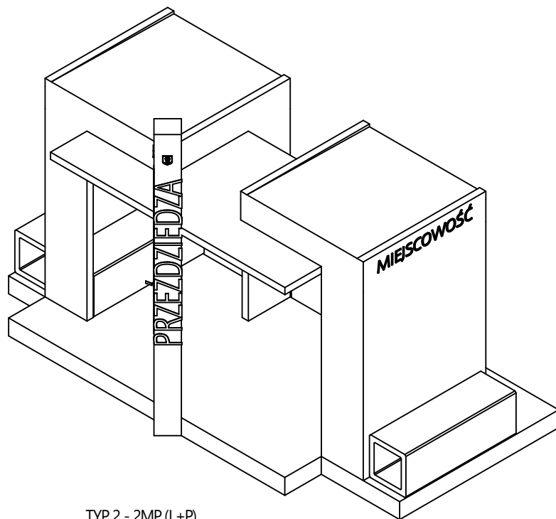
TYP 2 - 2MP (L+P) SŁUP Z ROZKŁADEM JAZDY +2 MODUŁY PODSTAWOWE
