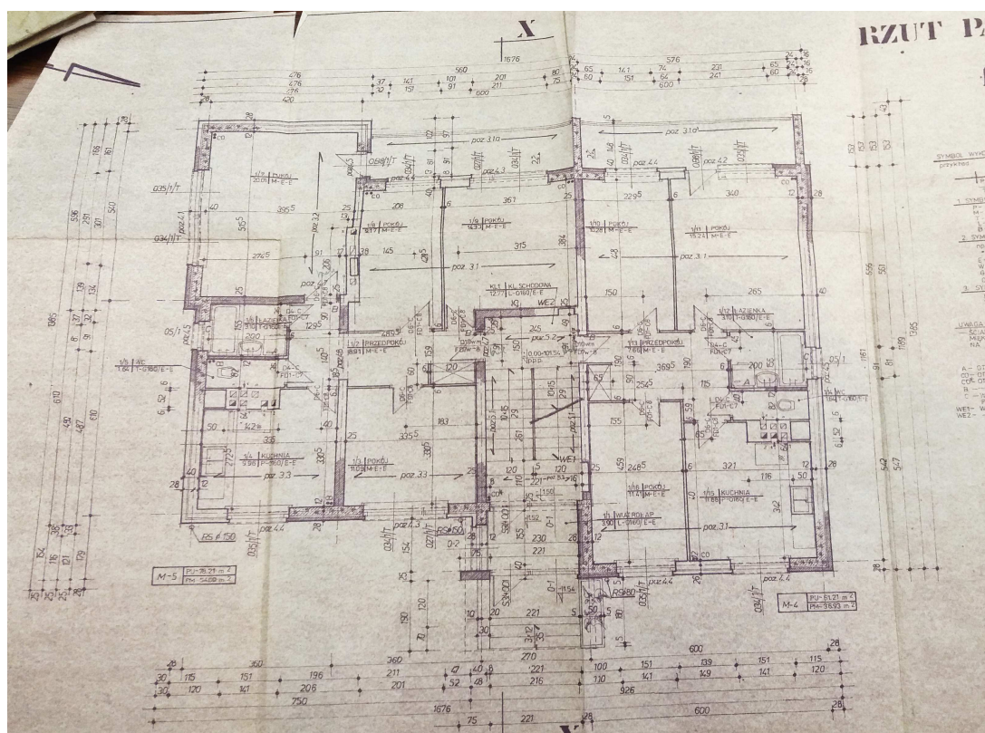
Rzut parteru
