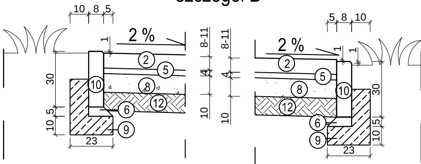
szczegół B
