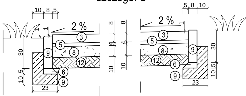
szczegół C
