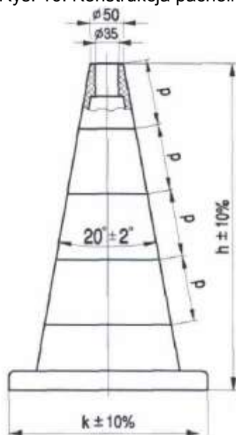
Rys. 10. Konstrukcja pachółki U-23 z wymiarami konstrukcyjnymi
