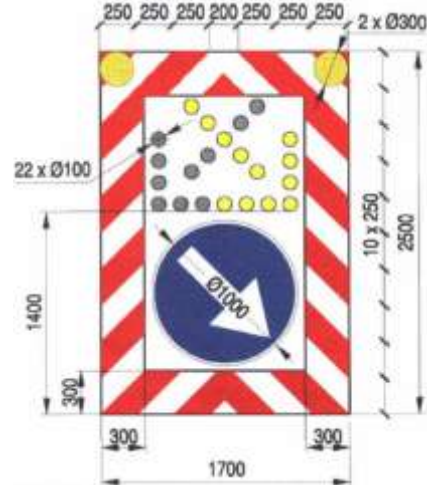
Rys. 17. Tablica zamykająca U-26c
