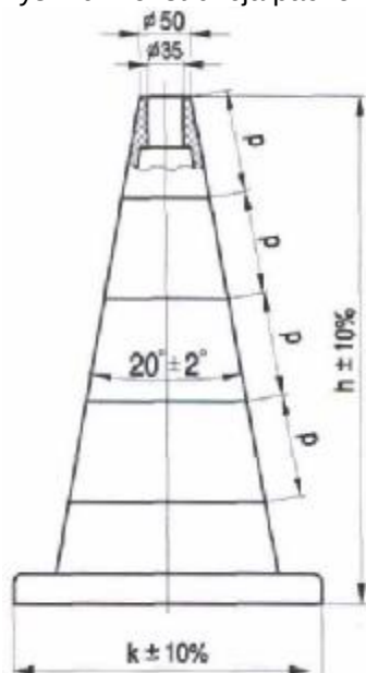
Rys. 10. Konstrukcja pachółka U-23 z wymiarami konstrukcyjnymi
