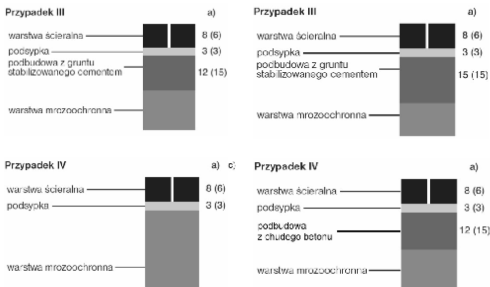
2.3. Konstrukcja nawierzchni dla kategorii ruchu R_2 – grubość warstwy w [cm]
