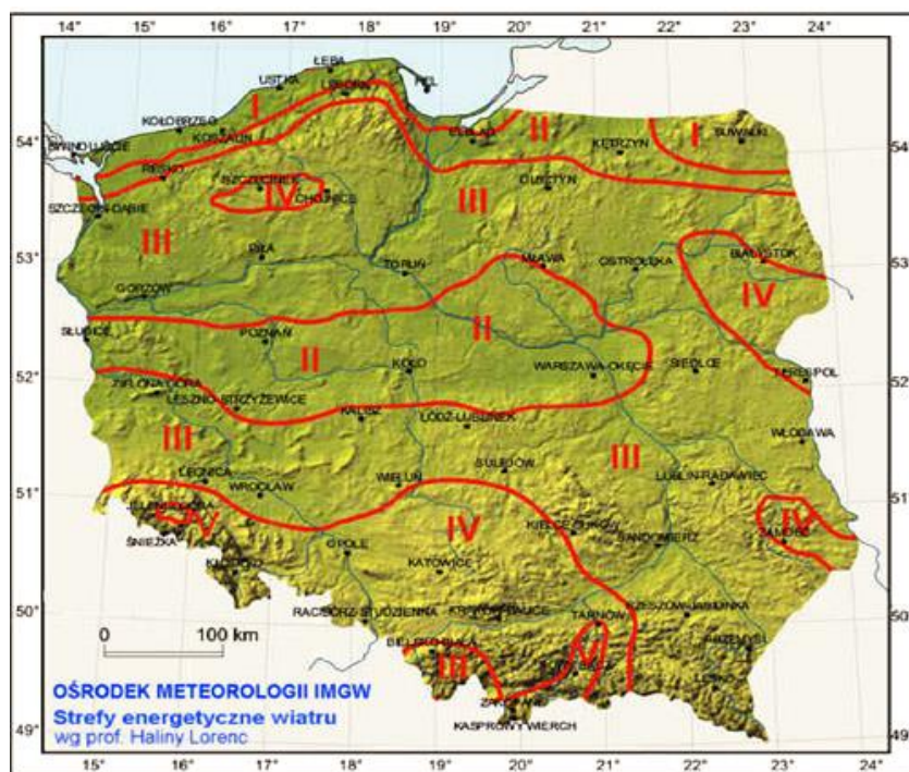
Rysunek 5. Strefy energetyczne wiatru w Polsce, (Źródło IMGW)
