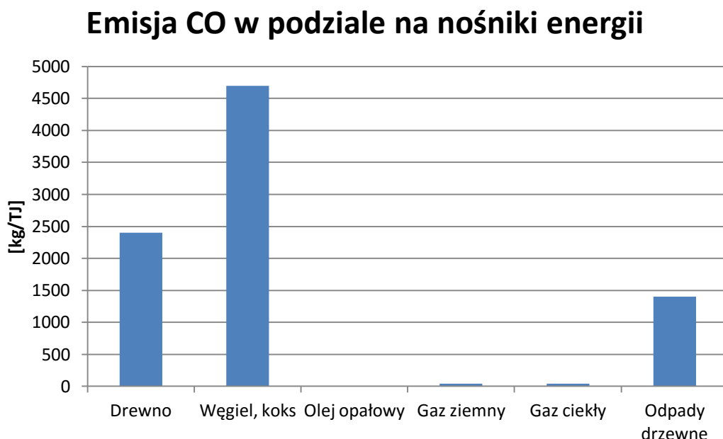
Wykres 4. Emisja CO w podziale na nośniki energii (wg: „Wskazówki dla wojewódzkich inwentaryzacji emisji na potrzeby ocen bieżących i programów ochrony powietrza”)
