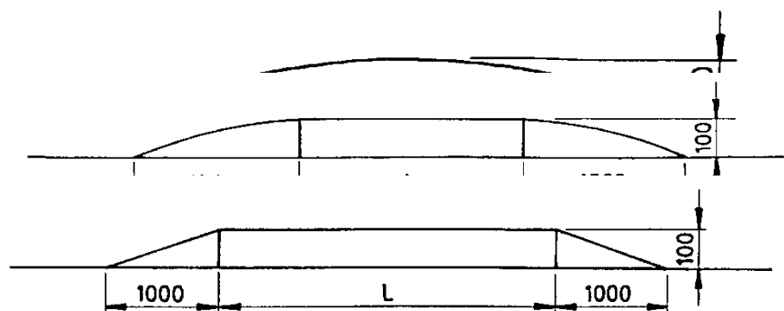
Rys. 1. Kształt i wymiary progów liniowych typu 1 (dla granicznej prędkości przejazdu 25-30 km/h)
