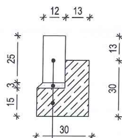
SZCZEGÓŁ A POSADOWIENIE OPORNIKA NA ŁAWIE BETONOWEJ SKALA 1:20
