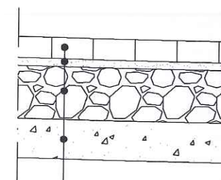
SZCZEGÓŁ G KONSTRUKCJA PROGU ZWALNIAJĄCEGO SKALA 1:20
