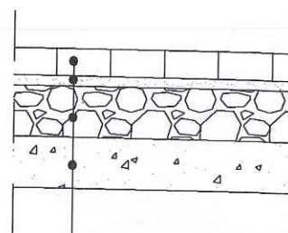
SZCZEGÓŁ E KONSTRUKCJA ZJAZDU SKALA 1:20
