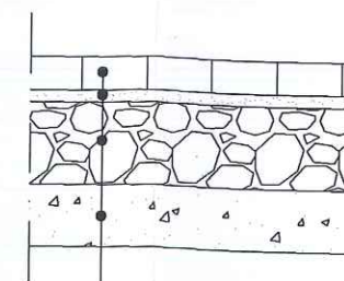
SZCZEGÓŁ D KONSTRUKCJA JEZDNI SKALA 1:20
