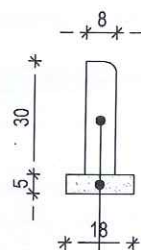
SZCZEGÓŁ B POSADOWIENIE OBRZEŻA NA PODSYPCE CEM-PIAS SKALA 1:20
