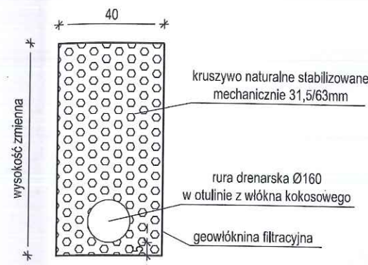
SZCZEGÓŁ C DREN FRANCUSKI SKALA 1:20
