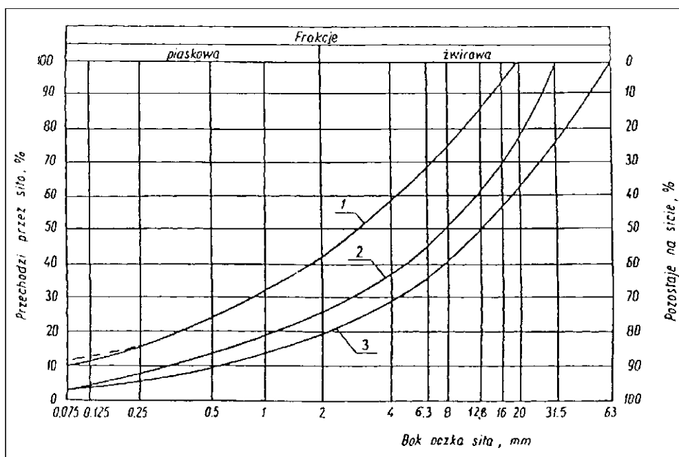
Rysunek 1. Pole dobrego uziarnienia kruszyw przeznaczonych na podbudowy wykonywane metodą stabilizacji mechanicznej 1-2 kruszywo na podbudowę zasadniczą (górną warstwę) lub podbudowę j jednowarstwową 1-3 kruszywo na podbudowę pomocniczą (dolną warstwę)
