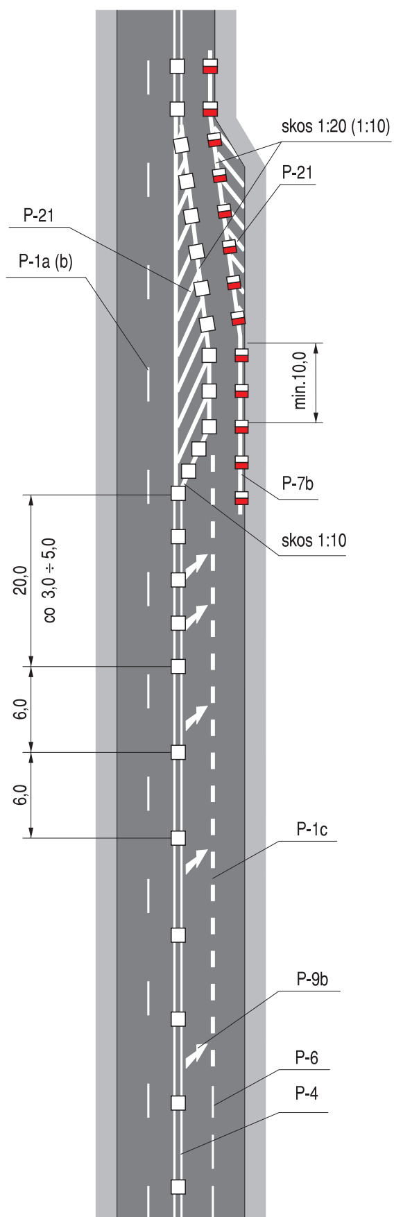
Rys. 6.3.3. Oznakowanie punktowymi elementami odbłaskowymi zanikającego pasa ruchu
