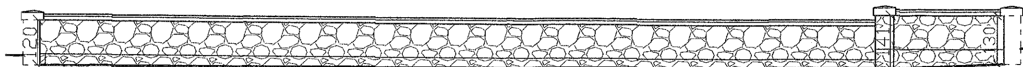
WIDOK CZĘŚCI WSCHODNIEJ OGRODZENIA OD STRONY WEWNĘTRZNEJ
