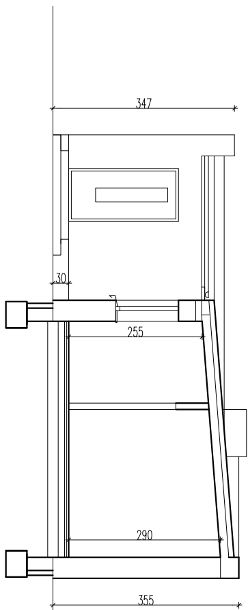
PRZEKRÓJ B-B
