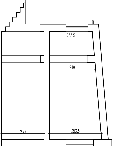
PRZEKRÓJ C-C
