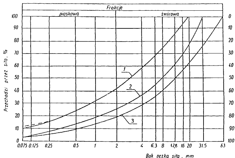
Rysunek 1. Pole dobrego uziarnienia kruszywa przeznaczonych na podbudowę wykonywane metodą stabilizacji mechanicznej 1-3 kruszywo na podbudowę pomocniczą (dolną warstwę)
