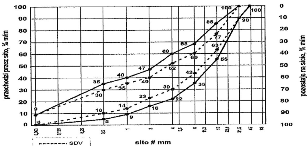
Rys. 1 Mieszanka niezwiązana 0/31 do warstw podbudowy zasadniczej
