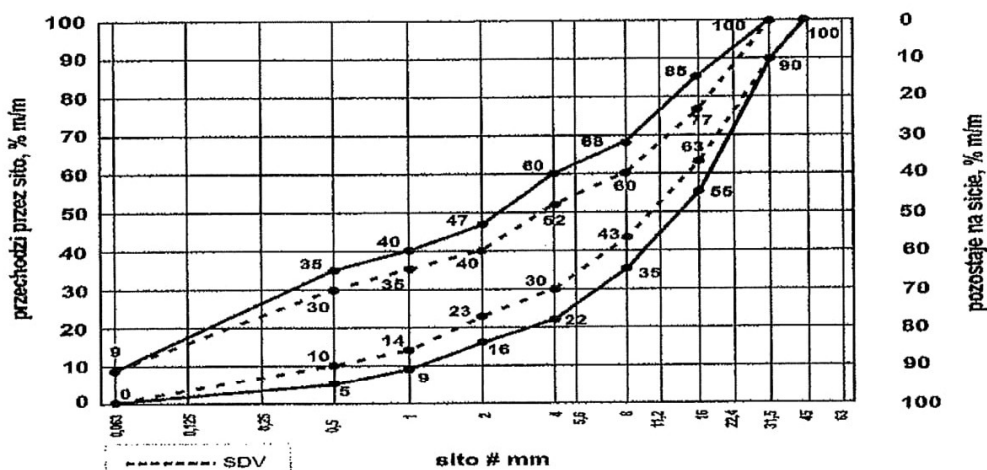
Rys. 1 Mieszanka niezwiązana 0/31 do warstw podbudowy zasadniczej
