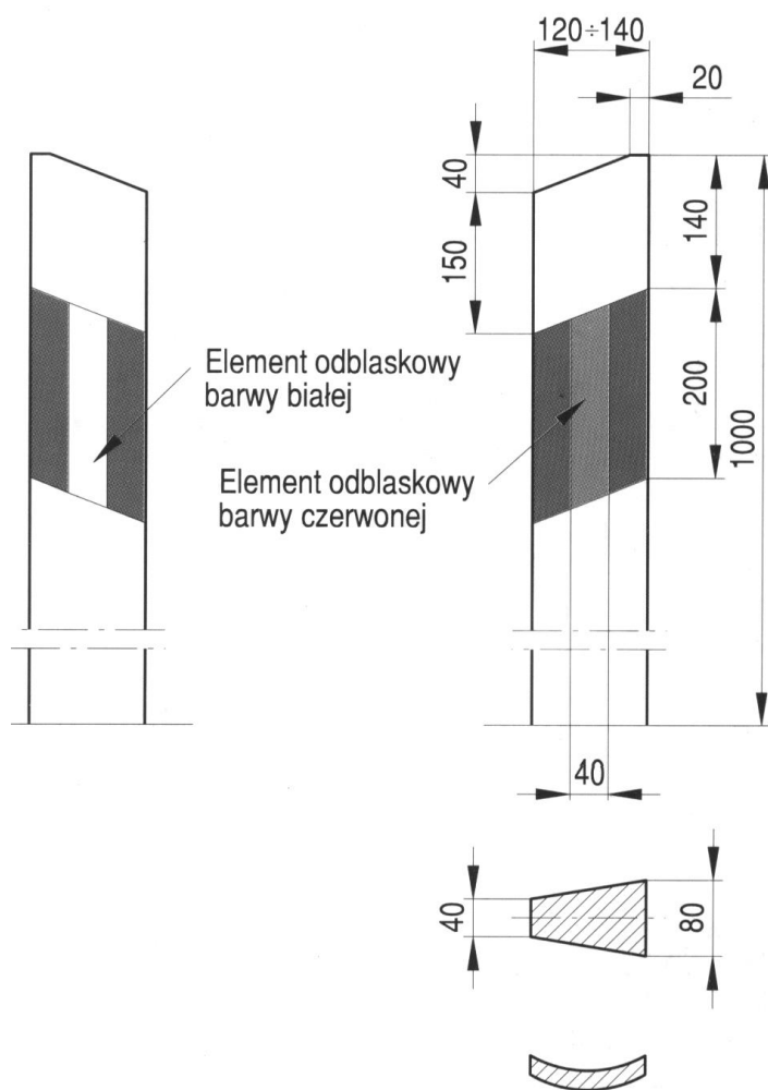
Rys. 1. Wzór słupka prowadzącego U-1a umieszczanych samodzielnie na poboczu.
