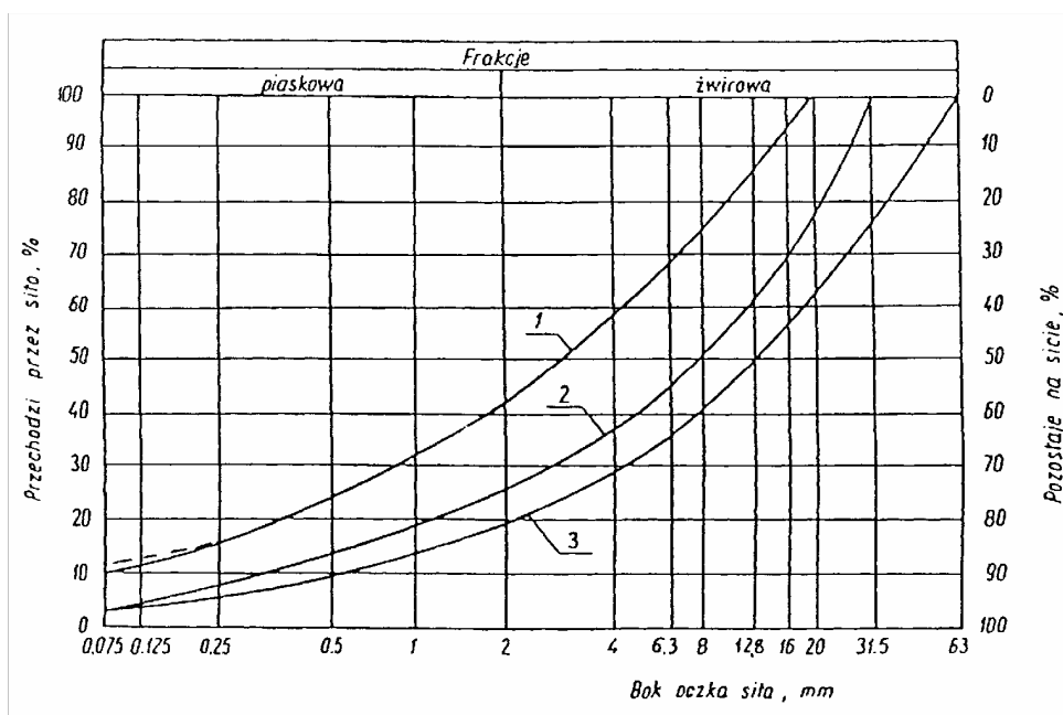
Rysunek 1. Pole dobrego uziarnienia kruszywa przeznaczonego na uzupełnianie poboczy 1-3 kruszywo na uzupełnienie poboczy
