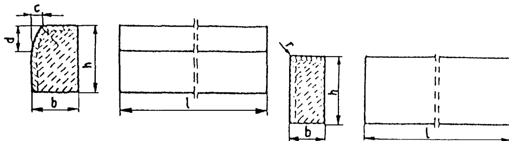
Rys. 1. Wymiarowanie krawężników
