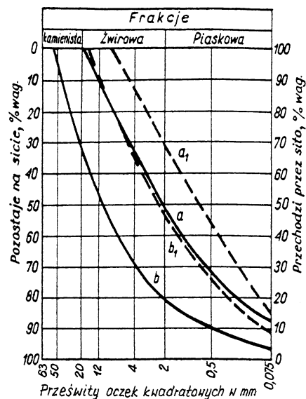
Rysunek 1. Obszar uziarnienia optymalnych mieszanek żwirowych
