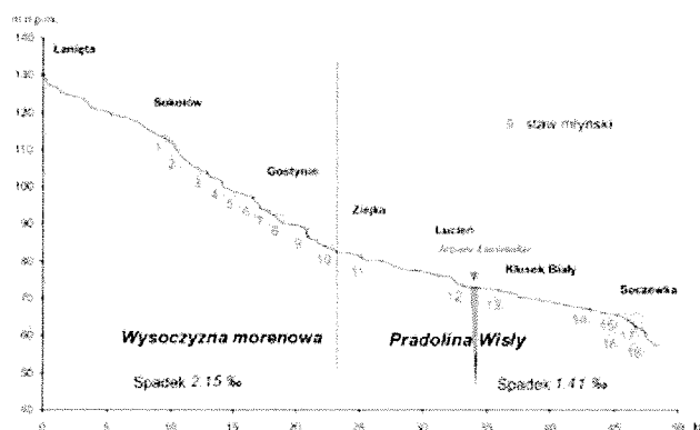
Profil podłużny rzeki Skrwy Lewej wraz z lokalizacją młynów wodnych
