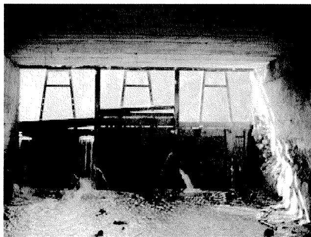
Zniszczony upust roboczy młyna wodnego Przerwa
