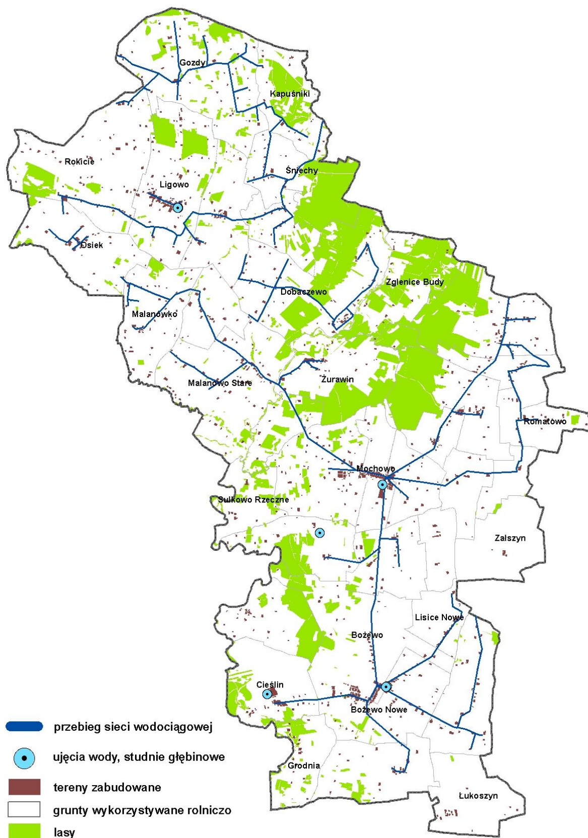
Ryc. 40 Schemat sieci wodociągowej w gminie Mochowo
