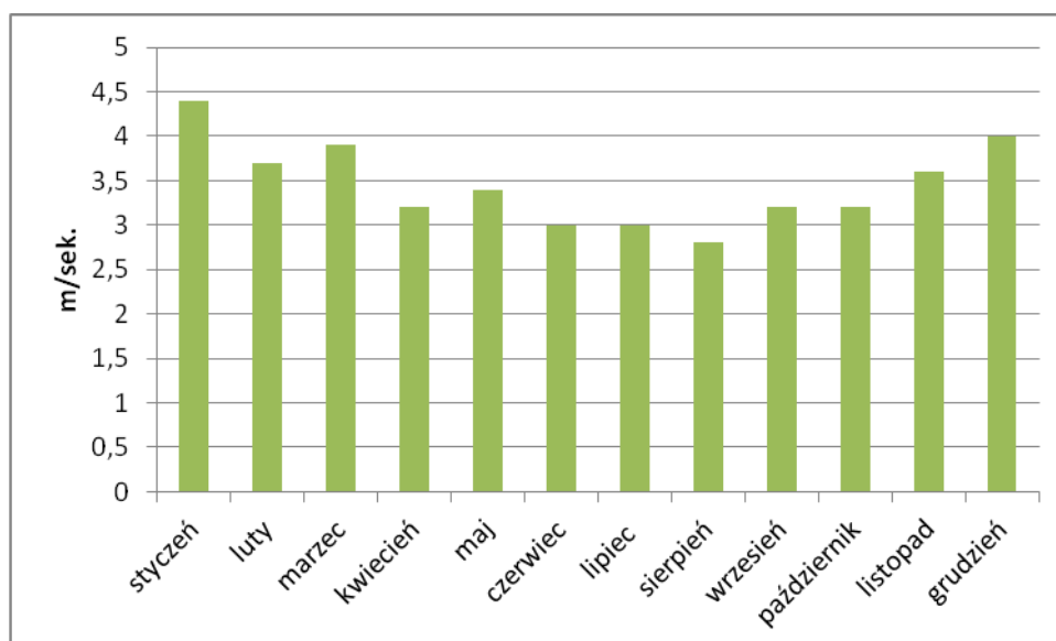
Ryc. 18 Średnia prędkość wiatru (m/sec.) dla stacji Płock Trzepowo.
