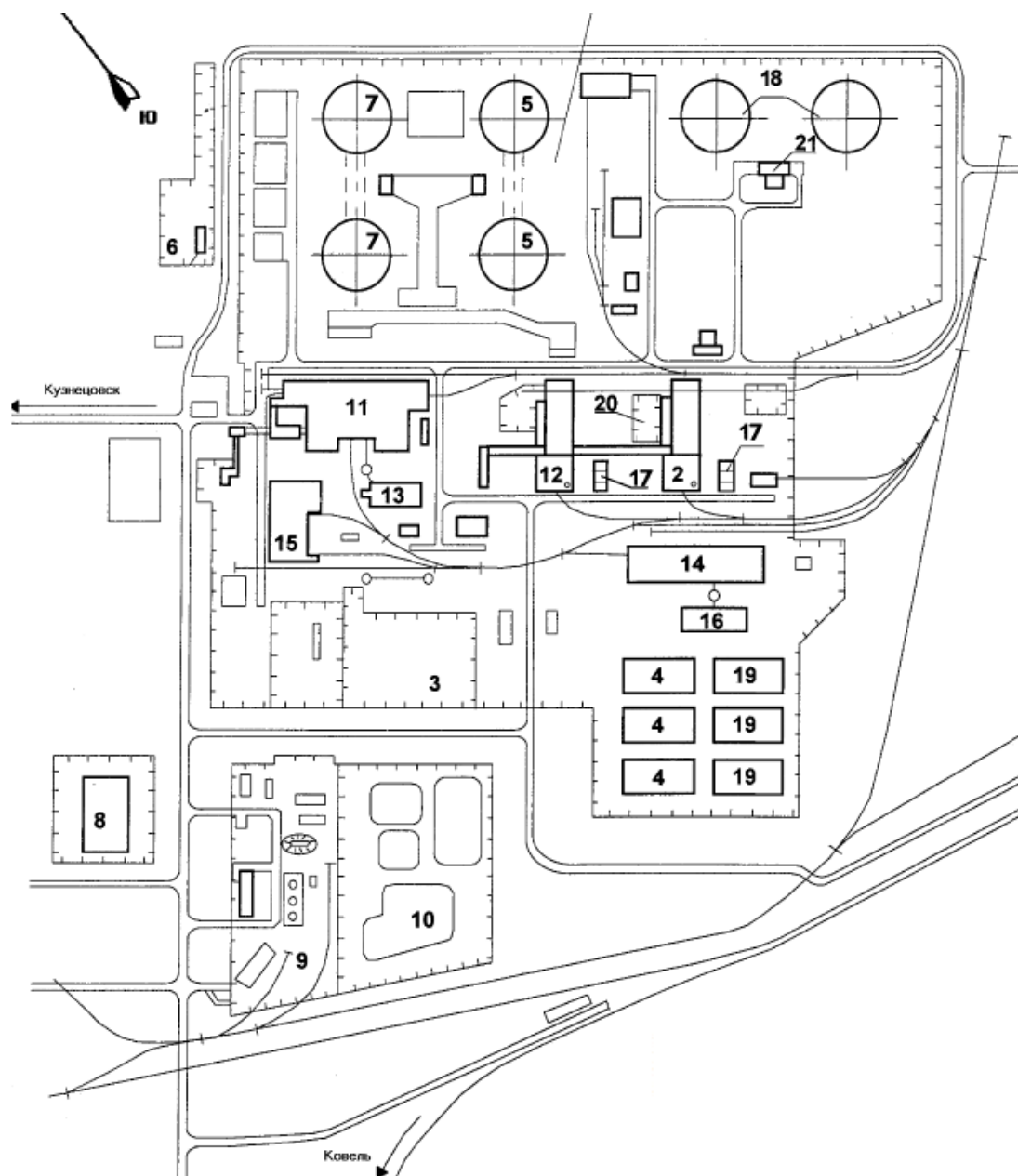
Rysunek 1.2 Schemat układu budynków i budowli na terenie przemysłowym SS Rówieńskij Elektrowni Jądrowej
