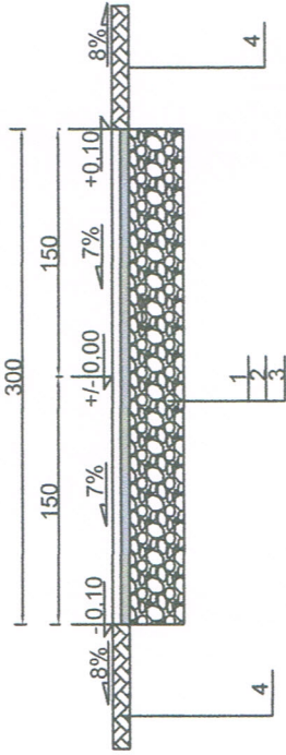
PRZEKRÓJ C – C
