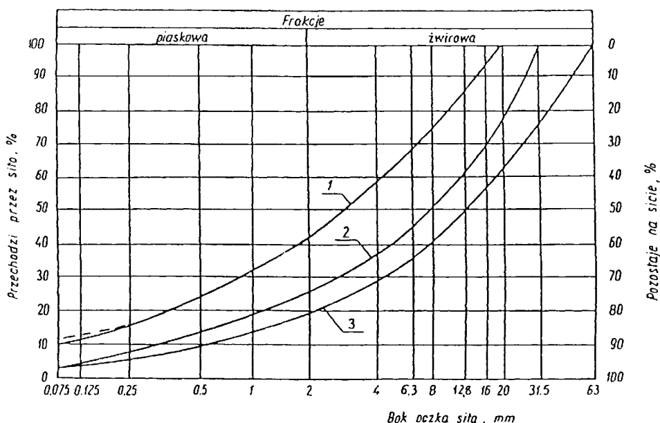
Rysunek 1. Pole dobrego uziarnienia kruszywa przeznaczonego na uzupełnianie poboczy
