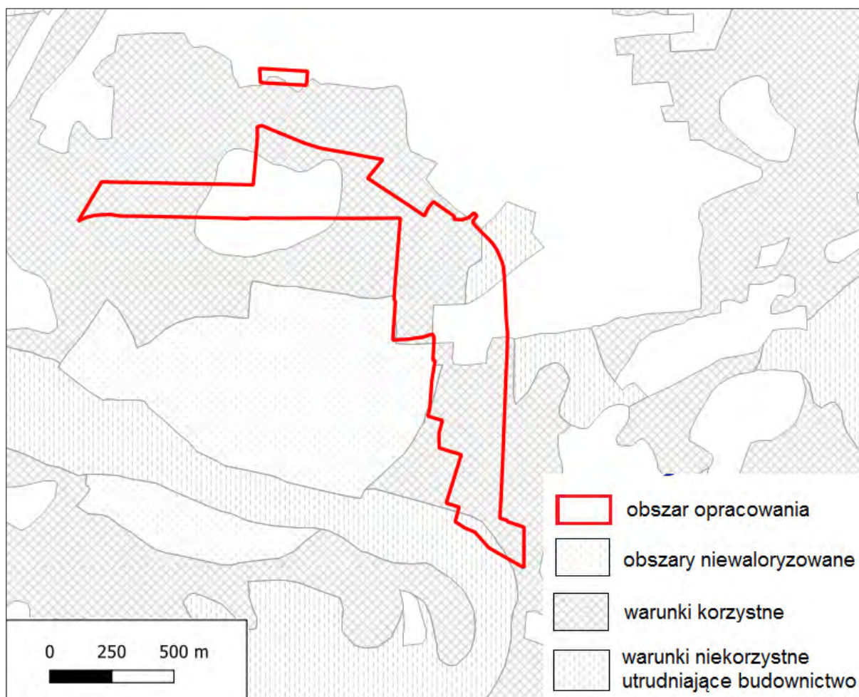
Rysunek 16 Warunki podłoża budowlanego na terenie A
