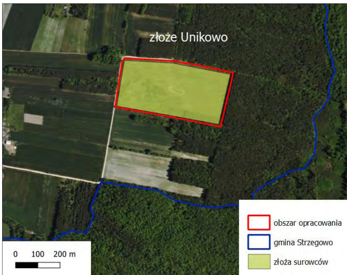
Rysunek 18. Występowanie złóż kopalin na terenie opracowania - B
