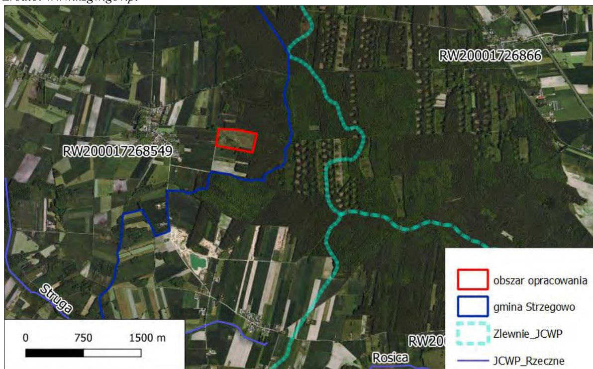
Rysunek 21. Mapa hydrologiczna z podziałem na zlewnie jednolitych części wód we fragmencie terenu Gminy Strzegowo wraz z zaznaczony terenem opracowania B Źródło: www.kzgw.gov.pl
