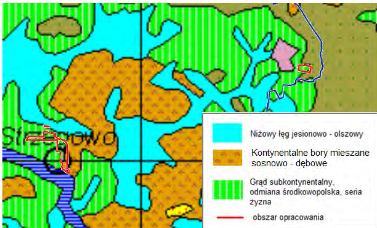
Rysunek 28. Potencjalna roślinność naturalna występująca we fragmencie Gminy Strzegowo Źródło: IGiPZ PAN, Warszawa
