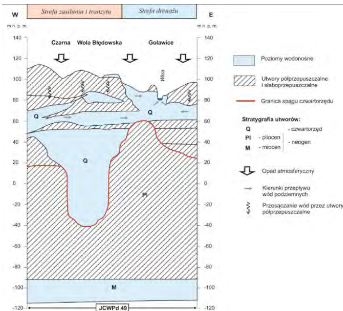
Rysunek 23. Schemat przepływu wód podziemnych w JCWPd nr 49 Źródło: www.psh.gov.pl
