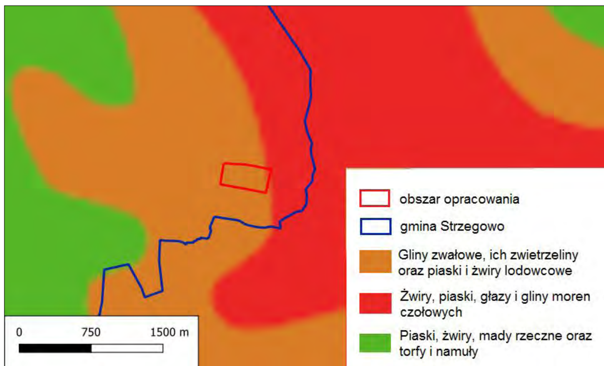
Rysunek 11. Mapa geologiczna fragmentu gminy Strzegowo wraz z zaznaczonym terenem B Źródło: http://m.bazagis.pgi.gov.pl/
