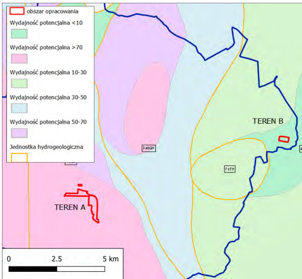
Rysunek 24 Wydajność potencjalna studni wierconej we fragmencie gminy Strzegowo wraz z zaznaczonym obszarem opracowania A i B Źródło: www.epsh.pgi.gov.pl/
