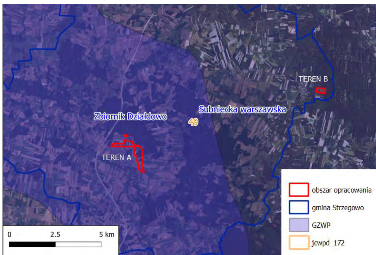
Rysunek 22. Położenie obszaru opracowania A i B na tle Głównych Zbiorników Wód Podziemnych oraz Jednolitych Części Wód Podziemnych
