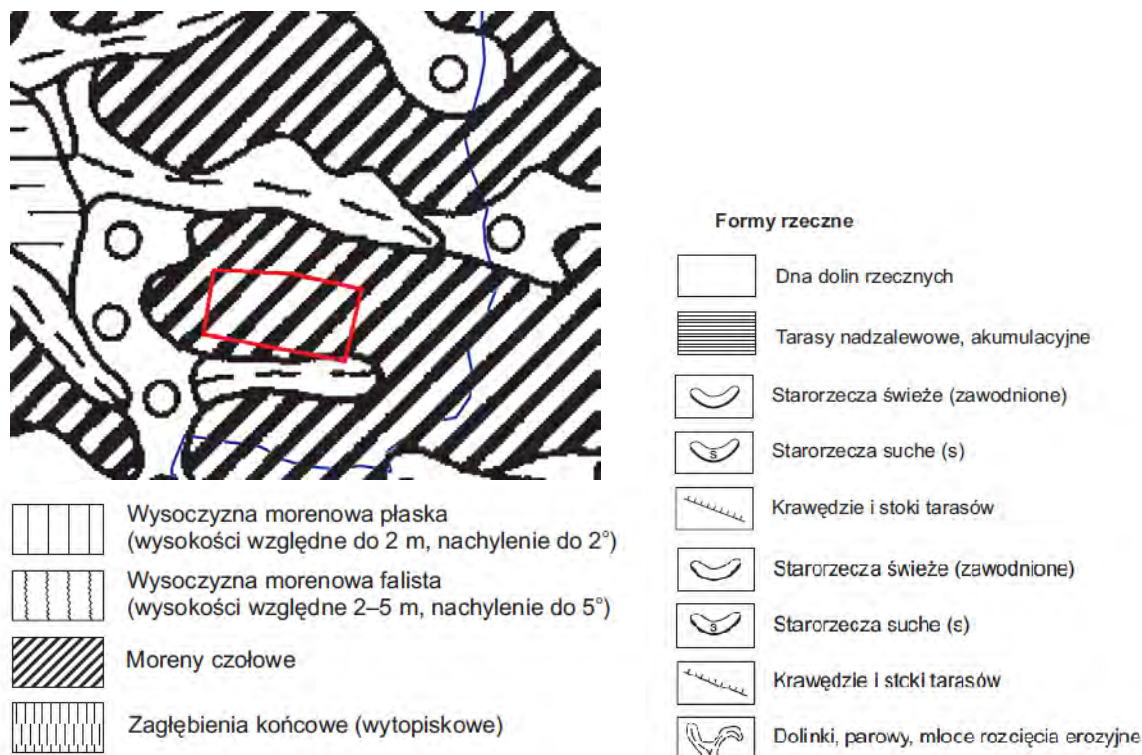
Rysunek 9. Szkic geomorfologiczny Skala 1:100 000 - teren B
