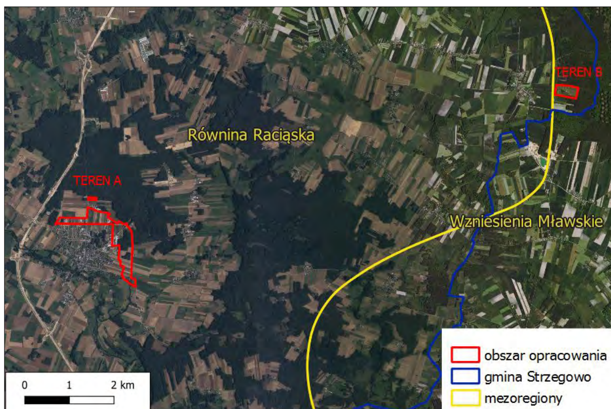
Rysunek 7. Obszar opracowania A i B na tle mezoregionów fizyczno-geograficznych Źródło: bazagis.pgi.gov.pl
