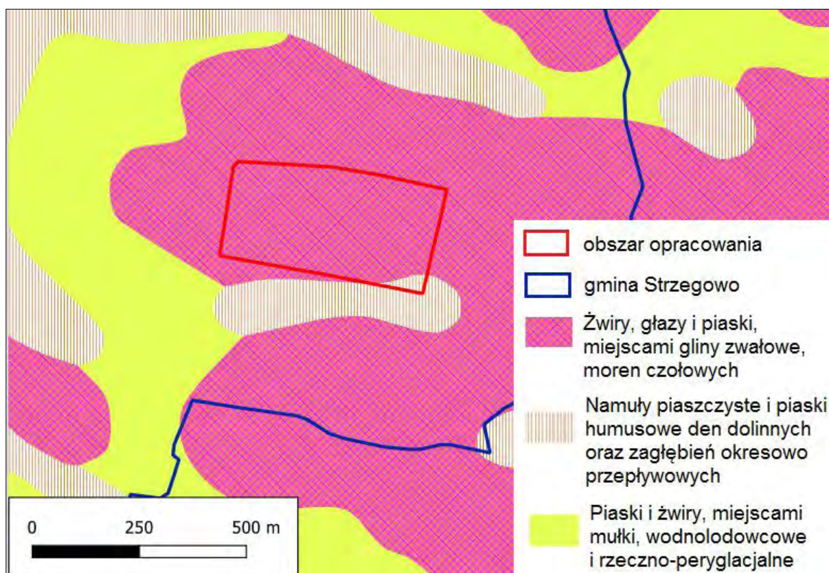
Rysunek 13. Fragment Szczegółowej Mapy Geologicznej Arkusz Strzegowo - Osada (368) - teren B Źródło: PIG
