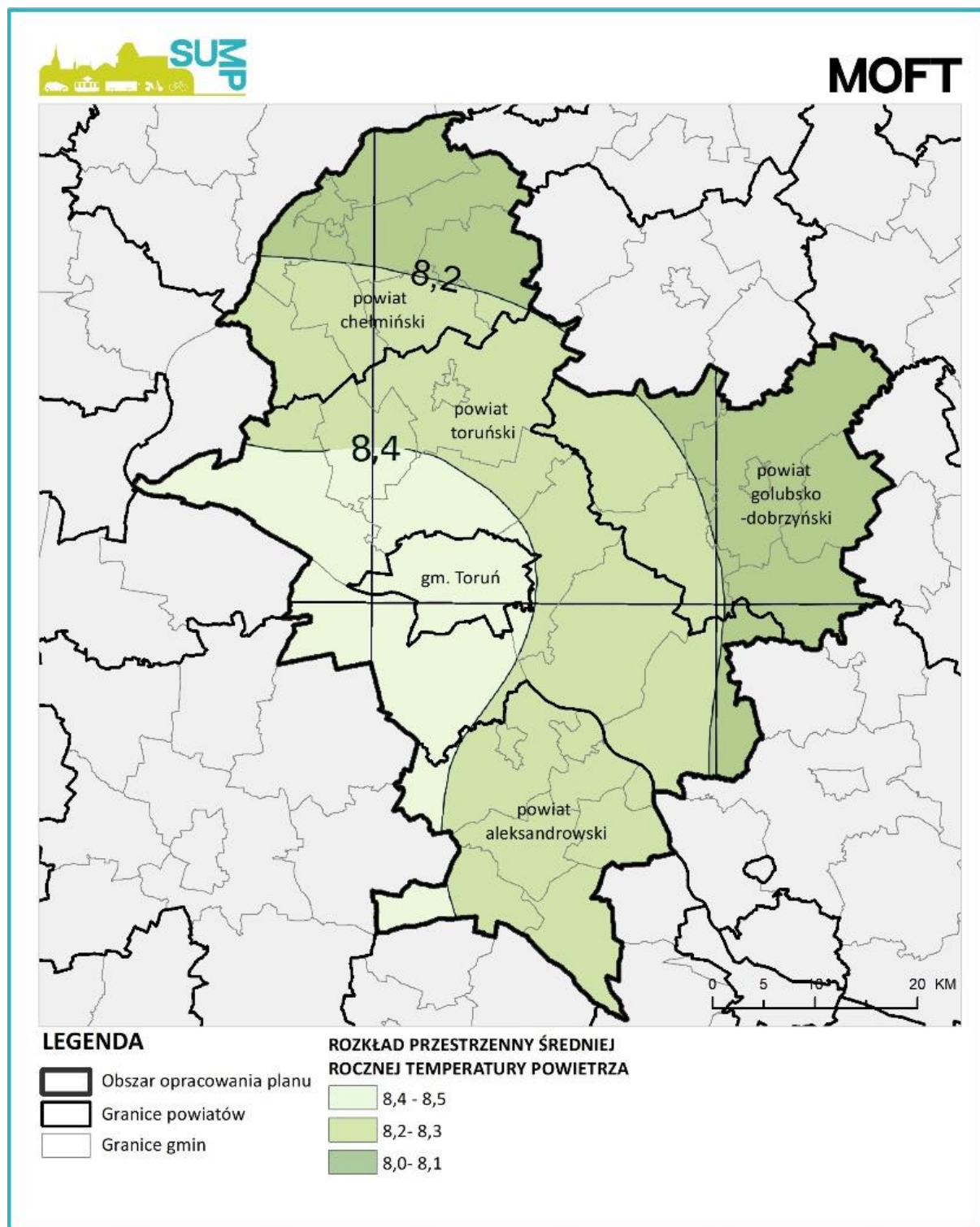
RYСУNEK 18. ROZKŁAD PRZESTRZENNY ŚREDNIEJ ROCZNEJ TEMPERATURY POWIETRZA.
