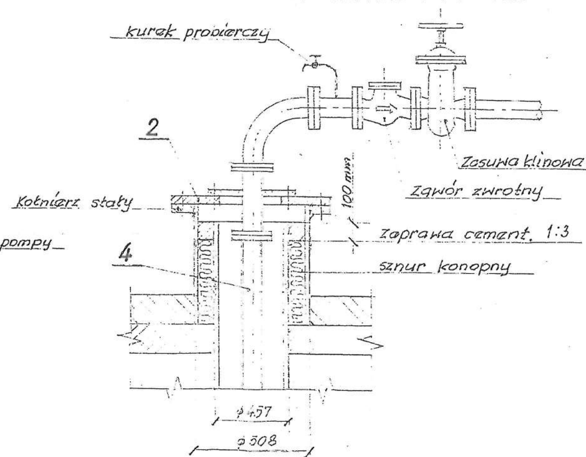
SCHEMAT UZBROJENIA INSTALACJI POMPWEJ
