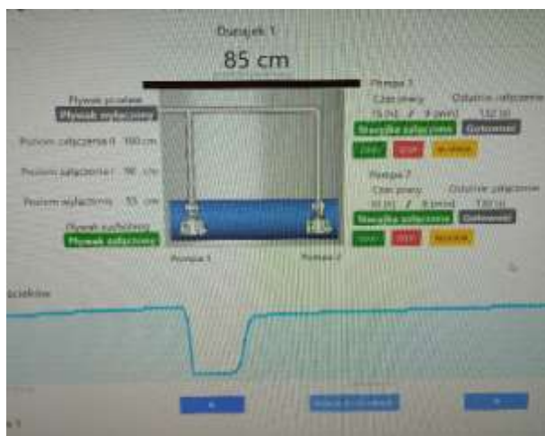
Podgląd na zmodernizowaną przepompownię w 2020 r.
