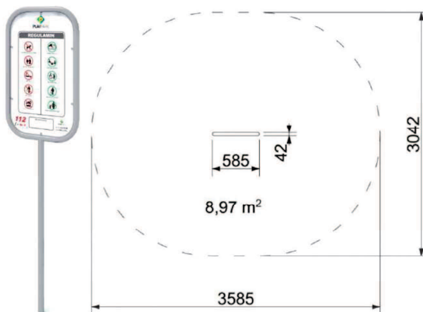
Rys. 11 Wymiary urządzenia
