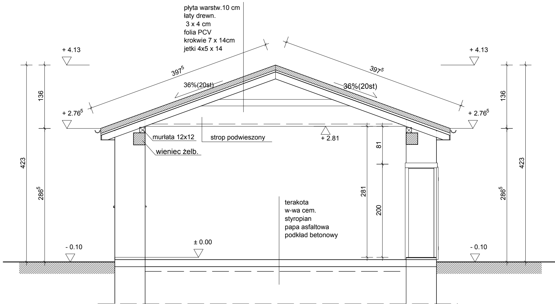
PRZEKRÓJ B-B
