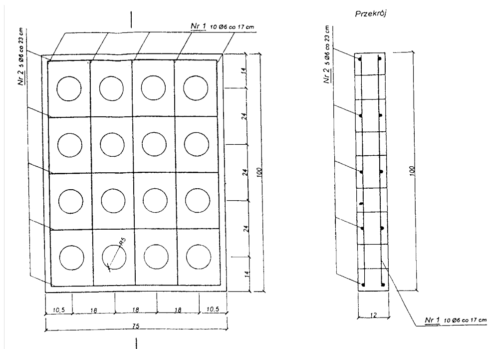
Rys. 2. Przykłady ułożenia płyt na jezdni jednopasowej
