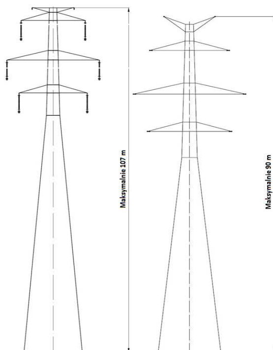
Ryc.11 Przykładowa sylwetka słupa przelotowego specjalnego, przykładowa sylwetka słupa mocnego M3 specjalnego
