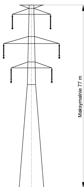
Ryc.9 Przykładowa sylwetka słupa przelotowego P
