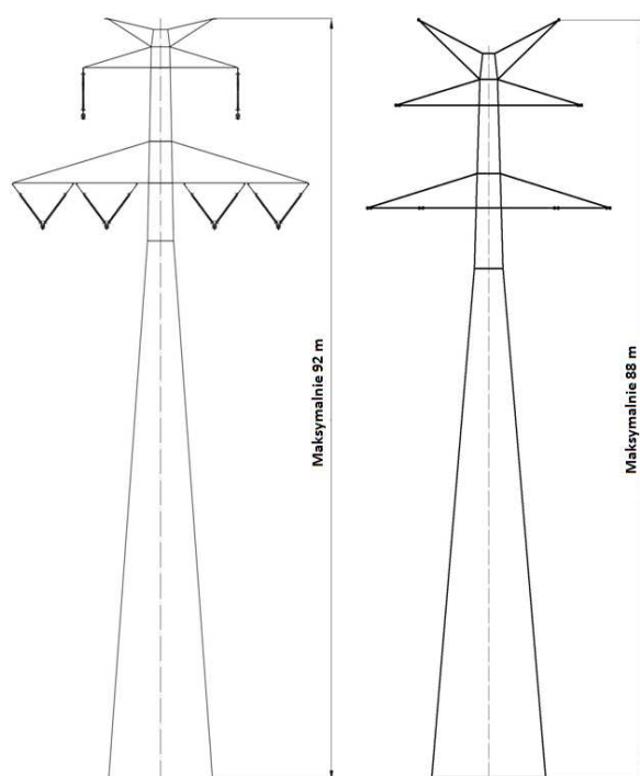
Ryc.10 Przykładowa sylwetka słupa przelotowego nadleśnego NPL, przykładowa sylwetka słupa mocnego nadleśnego
