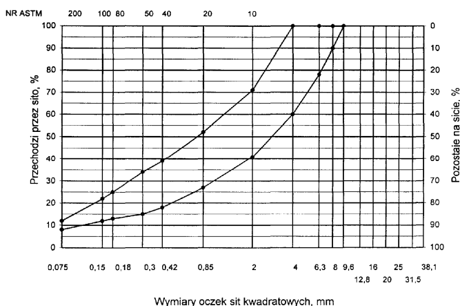
Rys. 1. Krzywe graniczne uziarnienia mieszanki mineralnej BA od 0 do 16mm, do warstwy ścieralnej nawierzchni drogi o obciążeniu ruchem KR2
