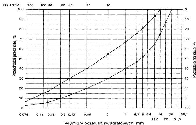
Rys. 2. Krzywe graniczne uziarnienia mieszanki mineralnej BA od 0 do 20 mm do warstwy wiążącej, wyrównawczej i wzmacniającej nawierzchni drogi o obciążeniu ruchem KR2
