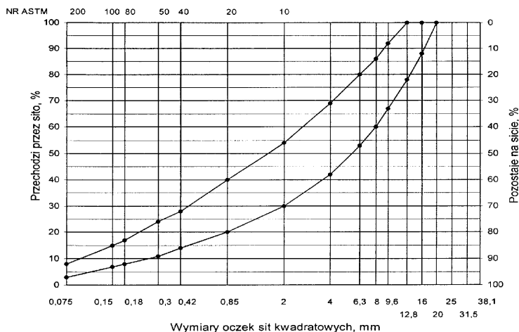
Rys. 4. Krzywe graniczne uziarnienia mieszanek mineralnych BA od 0 do 20 mm do warstwy wiążącej, wyrównawczej i wzmacniającej nawierzchni drogi o obciążeniu ruchem KR1 lub KR2
