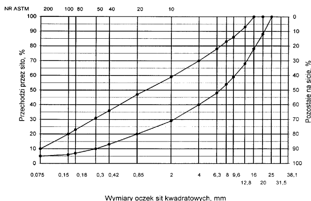
Rys. 1. Krzywe graniczne uziarnienia mieszanki min. BA od 0 do 20 mm do w-wy ścieralnej nawierzchni drogi o obciążeniu ruchem dla KR1 lub KR2
