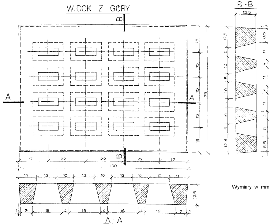
Rys. 1. Przykłady płyt żelbetonowych wielootworowych
